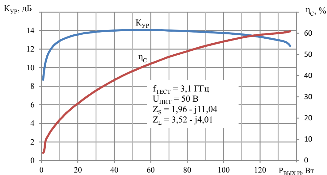
Рисунок 7. Типовая зависимость коэффициента усиления по мощности и коэффициента полезного действия стока от выходной импульсной мощности для транзистора ТНГ310100-50 на частоте 3,1 ГГц при t_k = (25 \pm 15)^\circ\text{C} и I_{c.0} = 100 мА
