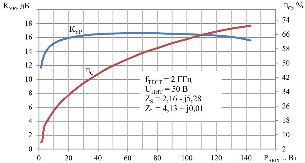
Рисунок 5. Типовая зависимость коэффициента усиления по мощности и коэффициента полезного действия стока от выходной импульсной мощности для транзистора ТНГ310100-50 на частоте 2 ГГц при t_k = (25 \pm 15) \text{ }^\circ\text{C} и I_{C.0} = 100 \text{ мА}
