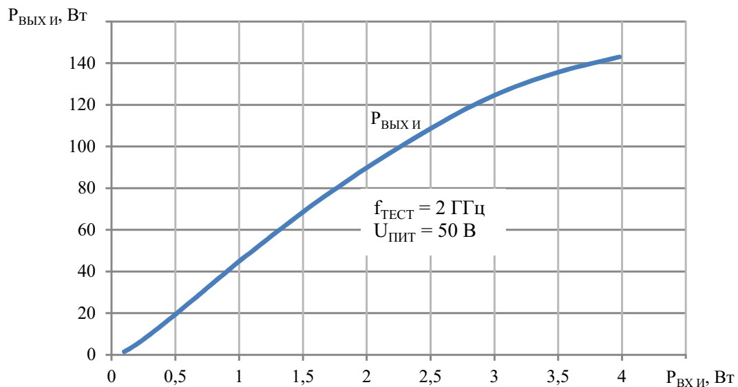
Рисунок 6. Типовая зависимость выходной импульсной мощности от входной импульсной мощности для транзистора ТНГ310100-50 на частоте 2 ГГц при t_k = (25 \pm 15) \text{ }^\circ\text{C} и I_{C.0} = 100 \text{ мА}
