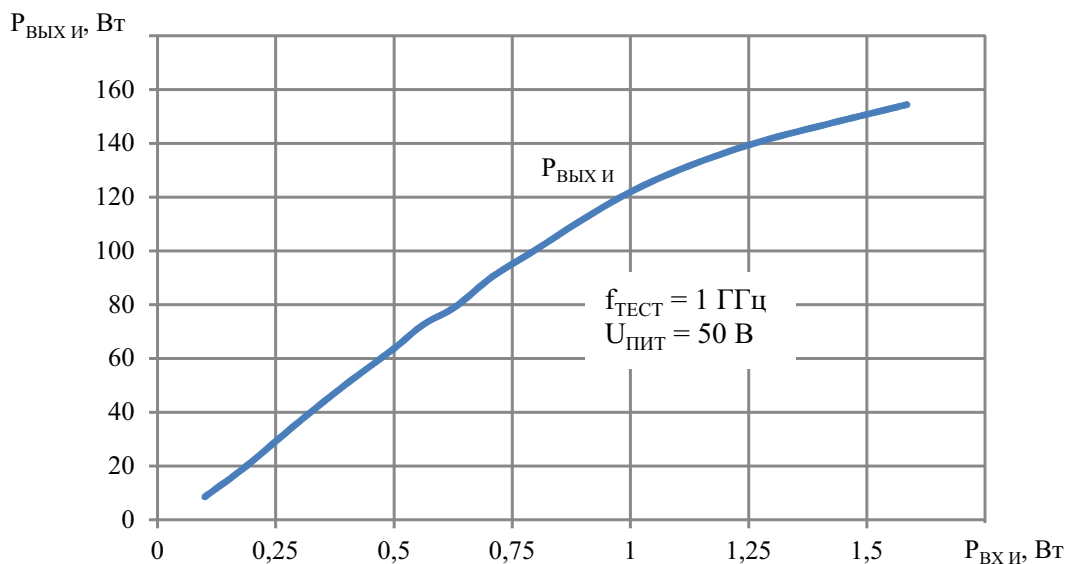
Рисунок 2. Типовая зависимость выходной импульсной мощности от входной импульсной мощности для транзистора ТНГ310100-50 на частоте 1 ГГц при t_{\kappa} = (25 \pm 15) \text{ }^\circ\text{C} и I_{\text{C.0.}} = 100 \text{ мА}
