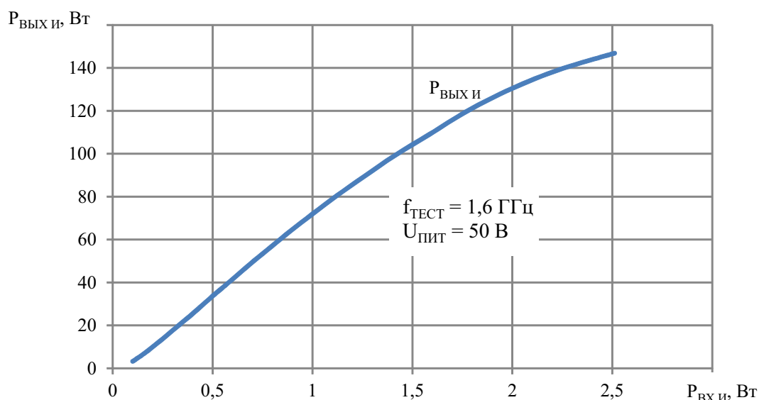
Рисунок 4. Типовая зависимость выходной импульсной мощности от входной импульсной мощности для транзистора ТНГ310100-50 на частоте 1,6 ГГц при t_k = (25 \pm 15)^\circ\text{C} и I_{C.0.} = 100 мА
