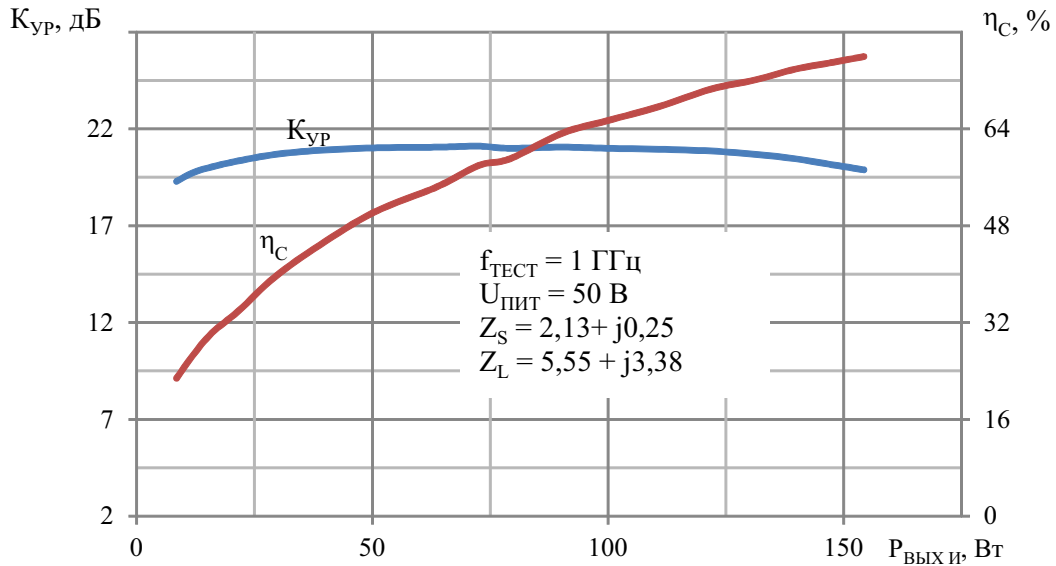
Рисунок 1. Типовая зависимость коэффициента усиления по мощности и коэффициента полезного действия стока от выходной импульсной мощности для транзистора ТНГ310100-50 на частоте 1 ГГц при t_{\kappa} = (25 \pm 15) \text{ }^\circ\text{C} и I_{\text{C.0.}} = 100 \text{ мА}
