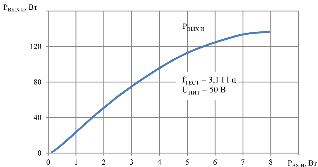
Рисунок 8. Типовая зависимость выходной импульсной мощности от входной импульсной мощности для транзистора ТНГ310100-50 на частоте 3,1 ГГц при t_k = (25 \pm 15)^\circ\text{C} и I_{c.0} = 100 мА
