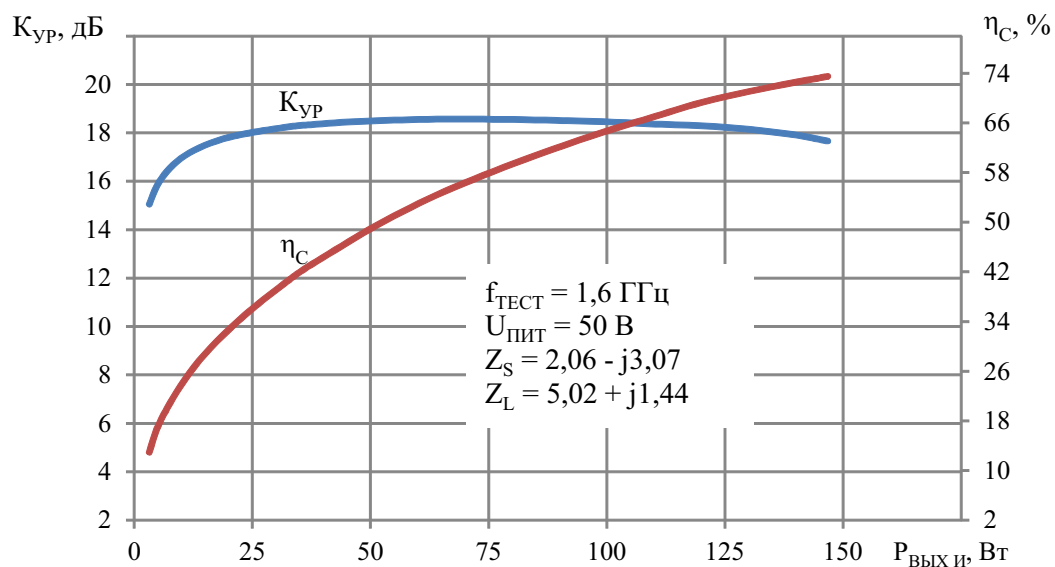
Рисунок 3. Типовая зависимость коэффициента усиления по мощности и коэффициента полезного действия стока от выходной импульсной мощности для транзистора ТНГ310100-50 на частоте 1,6 ГГц при t_k = (25 \pm 15)^\circ\text{C} и I_{C.0.} = 100 мА
